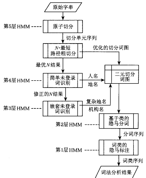
图 1 基于 CHMM 的汉语词法分析框架
