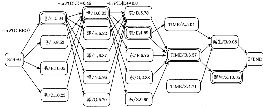
说明: ①图中节点的格式为: 词类 c_i / 角色 r_i , -\log P(c_i | r_i) , 双线结点 Viterbi 选优结果. ②图中的有向边权值为相邻角色的转移概率 -\log P(r_i | r_{i-1}) , 这里没有全部列出.
