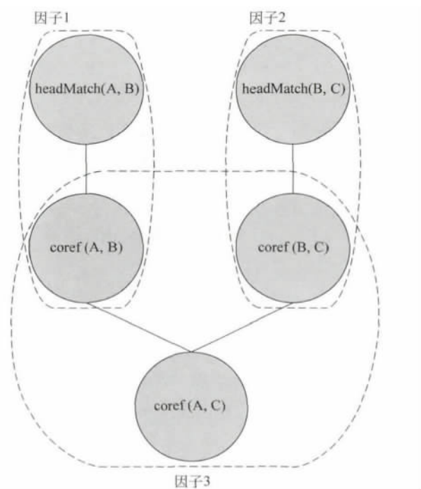
图1 根据公式(1),(2)和逻辑谓词 headMatch 生成的马尔科夫网络模型(其中虚线为马尔科夫图模型中的因子(factor))。
